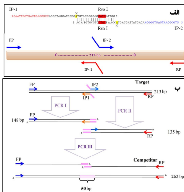
شکل 1- الف) آغازگرهای IP-1 و IP-2، ب) محصولات تولید شده در هر یک از واکنش‌های PCR I، PCR II، PCR III و PCR III Figure 1- A) Primers IP-1 and IP-2, B) PCR products in each reactions, PCRI, PCRII and PCRIII
