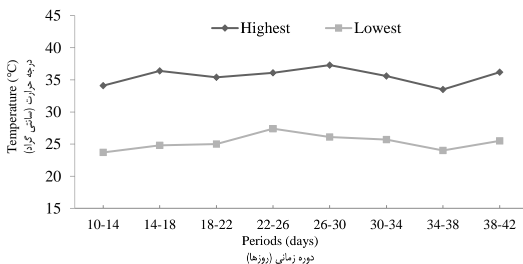
شکل ۱- درجه حرارت محیطی سالن آزمایشی
